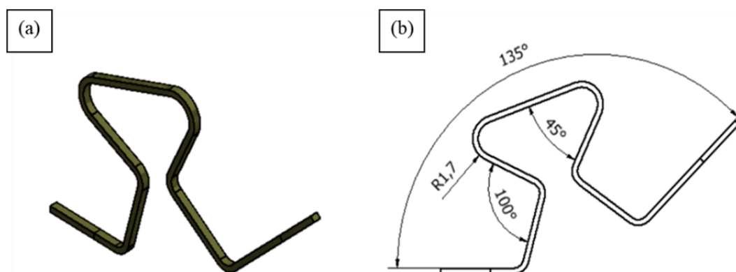
Fig. 1. (a) Modelo 3D da mola tipo T-loop ; (b) Dimensões principais.
