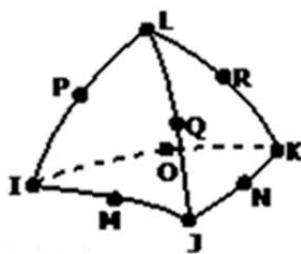
Fig. 3. Elemento tetraédrico de dez nós.
