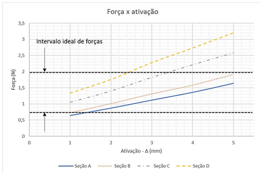
Fig. 5. Forças reativas.
