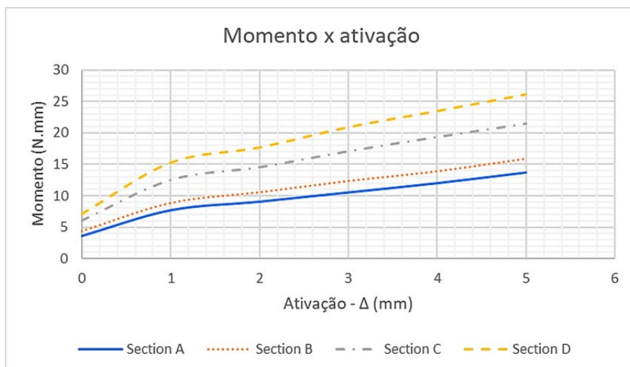
Fig. 6. Momentos reativos.
