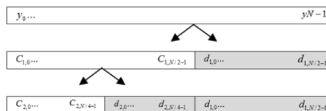
Fig. 4. Algoritmo piramidal para TWD.
