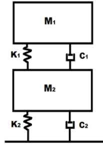
Fig. 5. Modelo dinâmico do edifício (Chavarette, Toniati, 2012).
