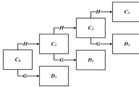
Fig. 3. Representação do algoritmo piramidal para TWD.
